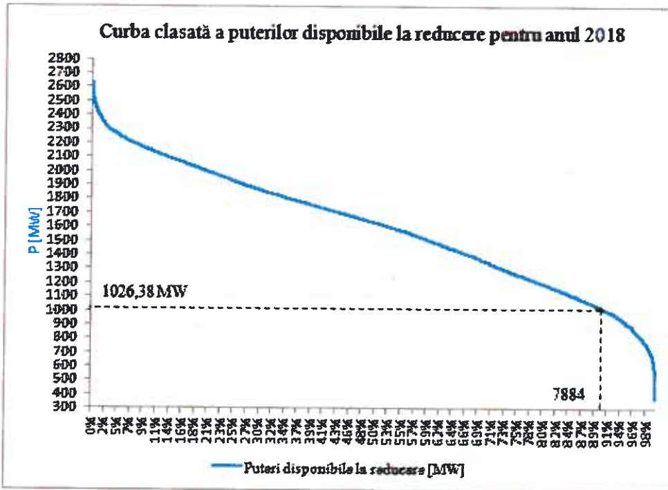
Fig. 1. Curba clasată a puterii active disponibilă la reducere, pe interval de o oră.
