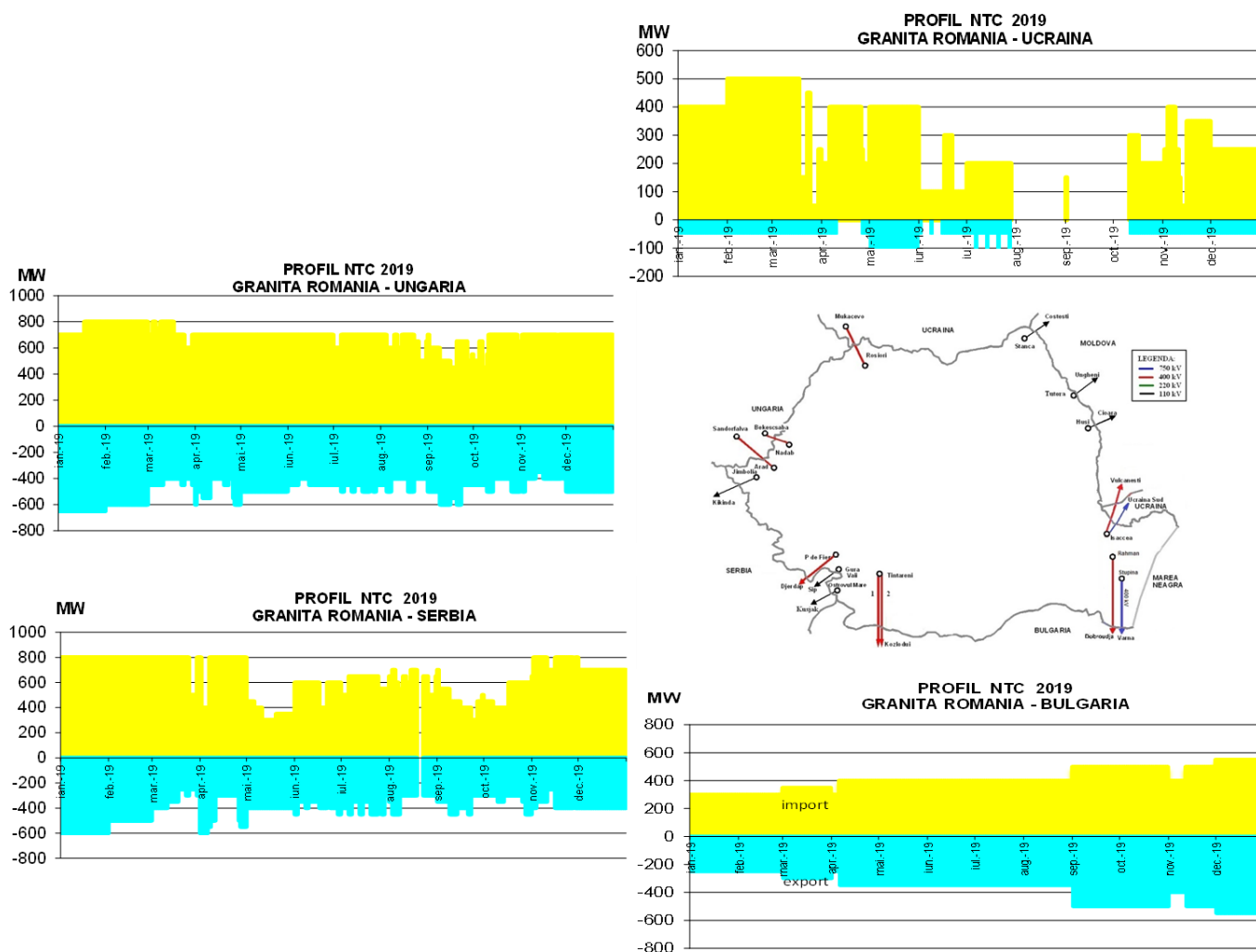
Fig. 2. Profilurile valorilor NTC pe granițe în anul 2019
