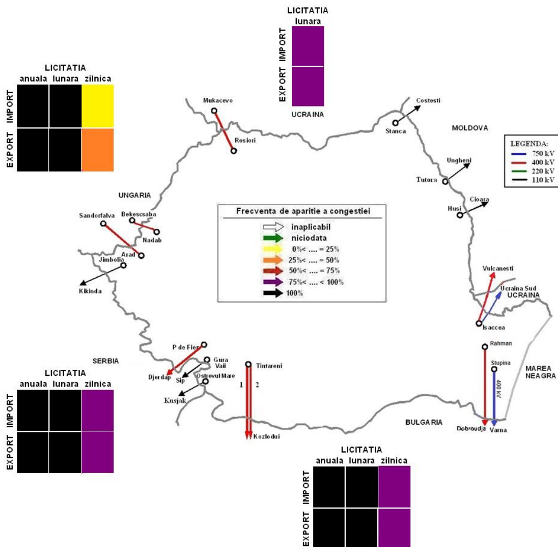
Fig. 1. Frecvența de apariție a congestiei în anul 2019
