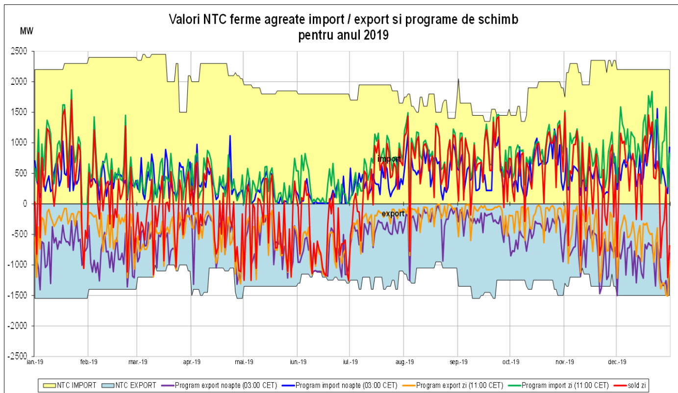
Fig. 3. Valori NTC ferme agreate și programe de schimb pentru anul 2019
