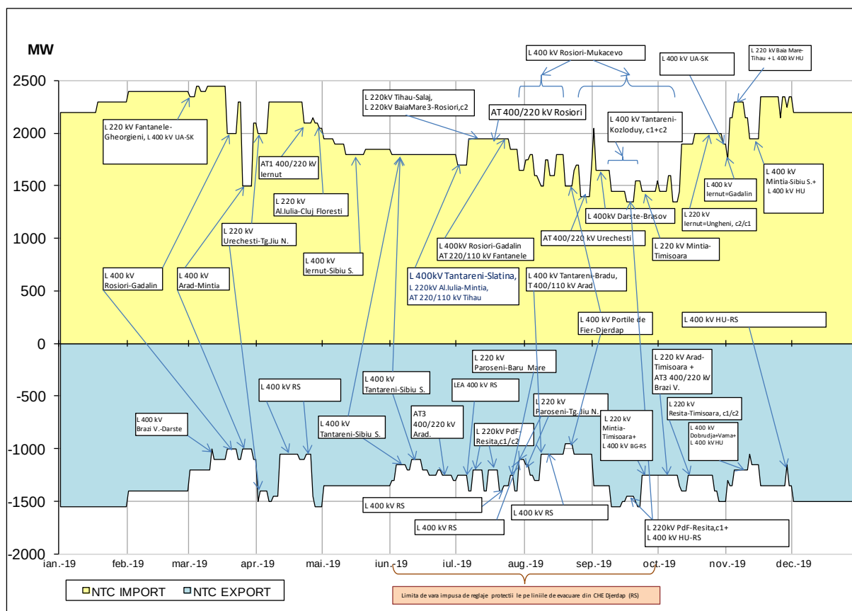
Fig. 5.4.4.2. Valori NTC ferme pentru import si export în anul 2019
