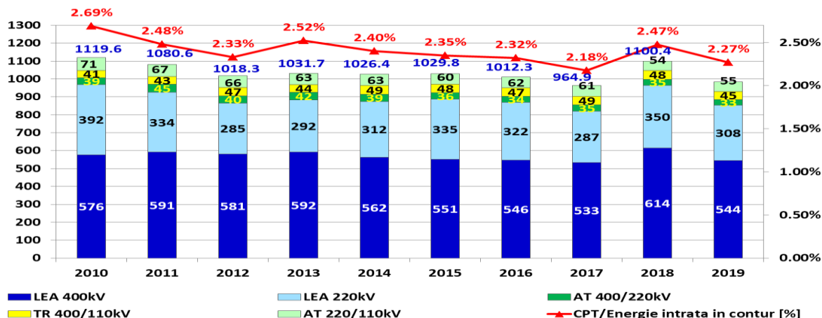
Evolutia anuală a CPT și a ponderii acestuia în energia intrată în contur
