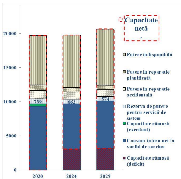
Fig. 9.5.2 Balanțe de putere - Analiza de sensibilitate (scenariul critic)
