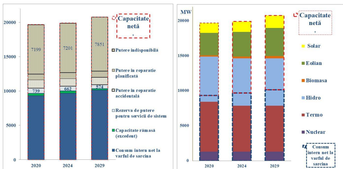
Fig. 9.5.1 Balanțe de putere - Scenariul de Referință
