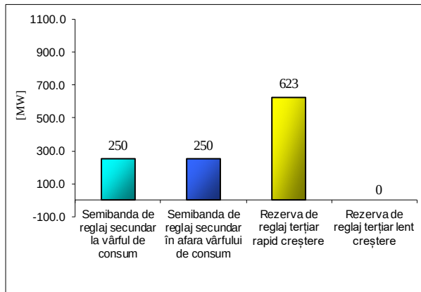
Cantități medii solicitate [hMW/h]
