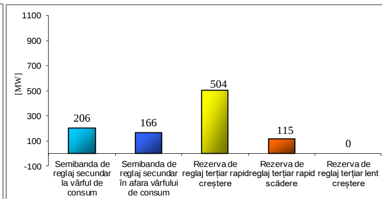
Cantități medii realizate [hMW/h]
