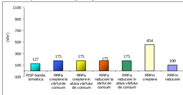
Cantități medii contractate [hMW/h]
