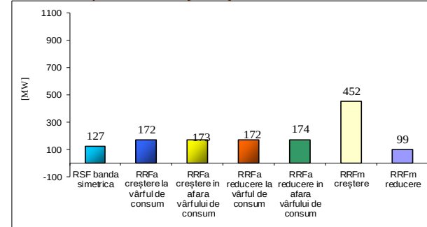
Cantități medii realizate [hMW/h]
