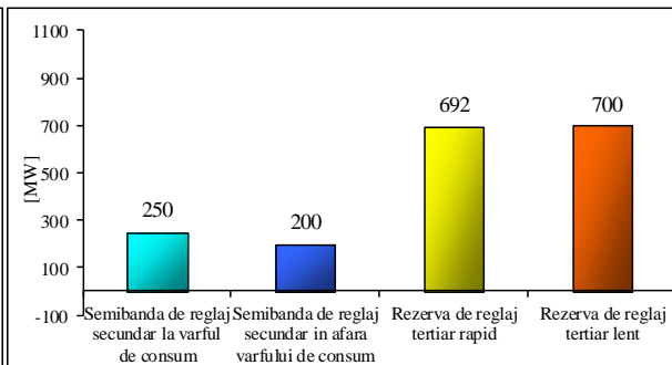
Cantitati medii contractate [hMW/h]
