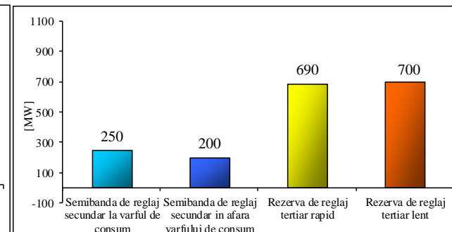
Cantitati medii realizate [hMW/h]
