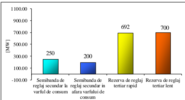
Cantitati medii solicitate [hMW/h]
