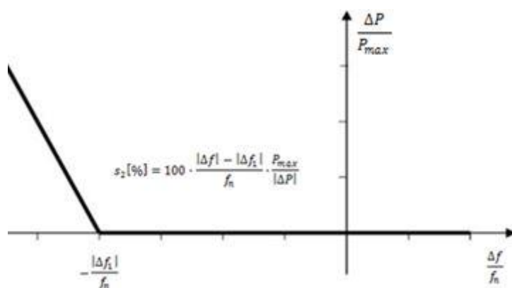
Fig. 3. Capabilitatea de răspuns la scăderea frecvenței a centralelor formate din module generatoare offshore (RFA-SC)
