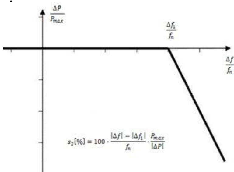
Fig. 1D. Capabilitatea de răspuns în putere activă la abaterile de frecvență în modul RFA-CR pentru centralele formate din module generatoare, de categorie D
