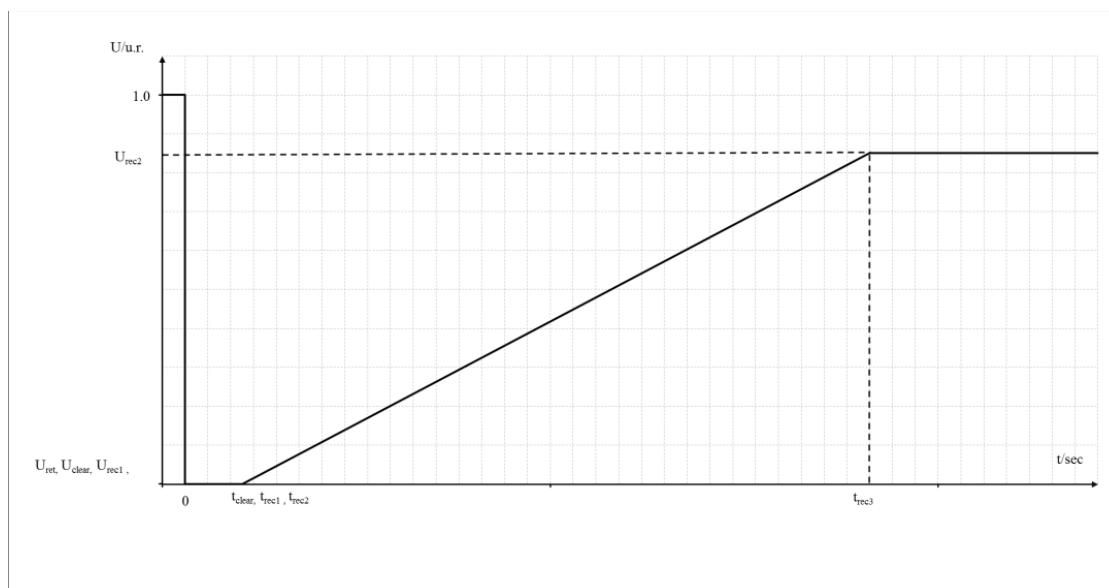
Fig. 6D. Diagrama de capabilitate privind trecerea peste defect a unui modul generator de categorie D
