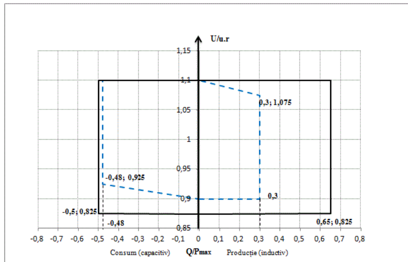
Fig. 7 Diagrama U-Q/P_{max} a unei centrale formată din module generatoare offshore
