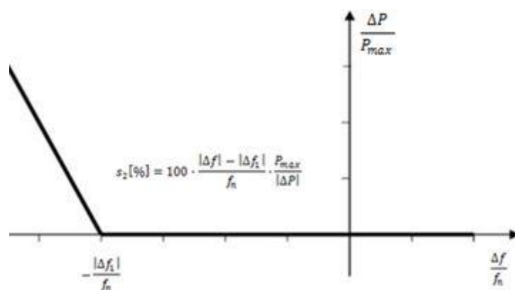
Fig. 3D. Capabilitatea de răspuns în putere activă la abaterile de frecvență în modul RFA-SC a centralelor formate din module generatoare, de categorie D
