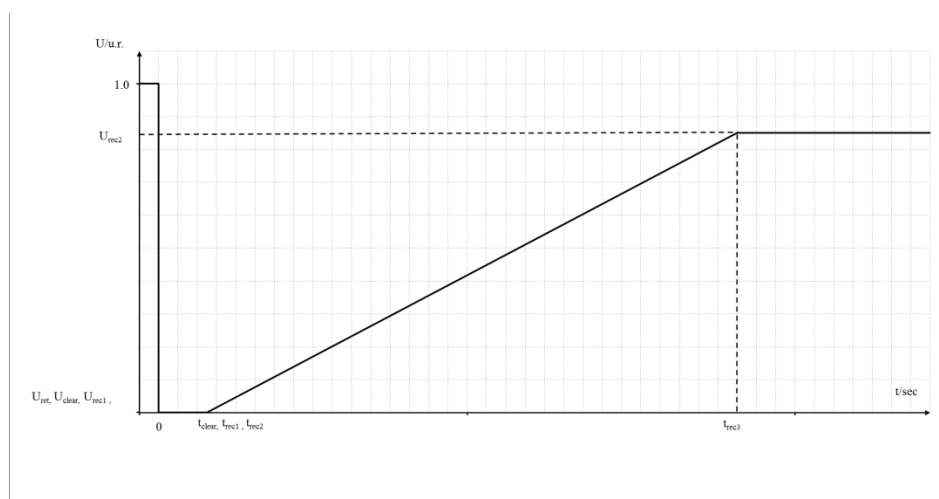
Fig. 6D. Diagrama de capacitate privind trecerea peste defect a unei centrale formate din module generatoare, de categorie D
