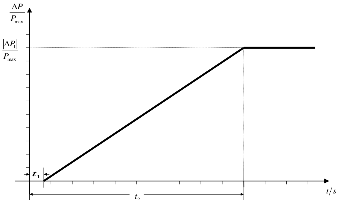
Fig. 5D. Capabilitatea de răspuns la abaterile de frecvență
