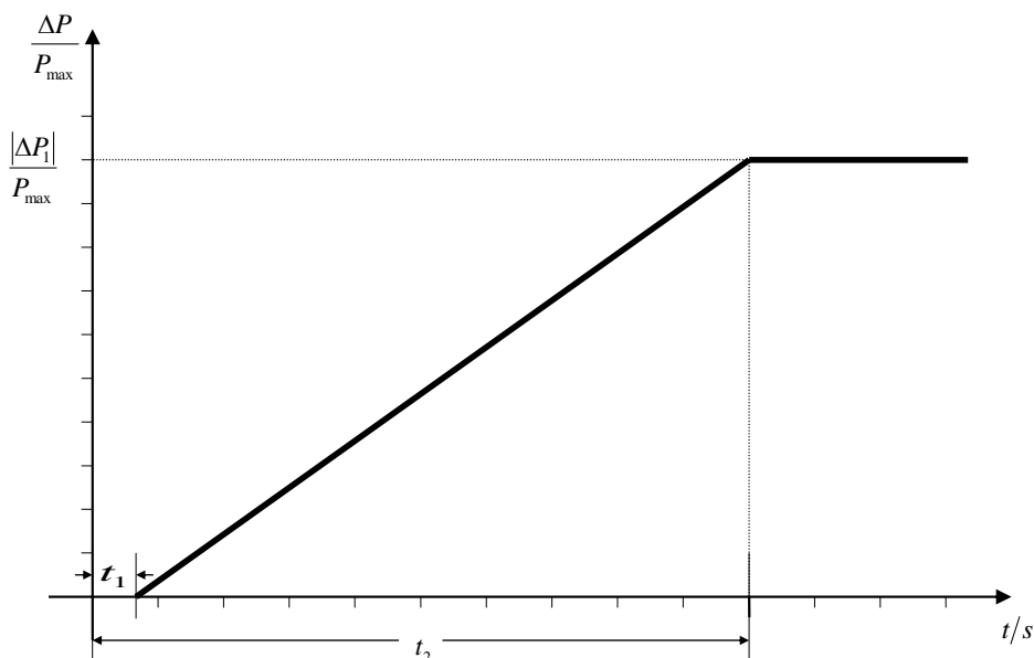
Fig. 5. Capabilitatea de răspuns la abaterile de frecvență
