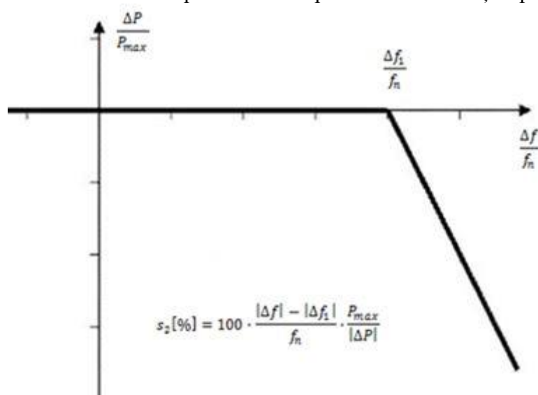
Fig. 1D. Capabilitatea de răspuns în putere activă la abaterile de frecvență în modul RFA-CR pentru modulele generatoare de categorie D
