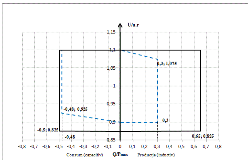
Fig. 7D. Diagrama U-Q/P_{\max} a unei centrale cu module generatoare
