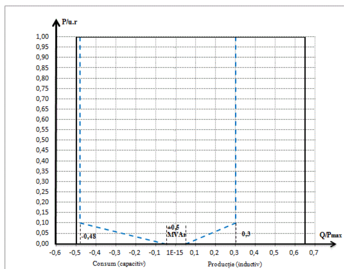
Fig. 8. Diagrama P-Q/P_{max} a unei centrale formată din module generatoare offshore
