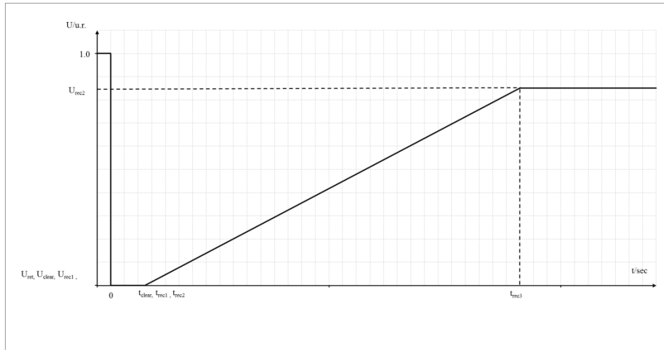
Fig. 6.1. Diagrama de capabilitate privind trecerea peste defect a unei centrale formată din module generatoare offshore
