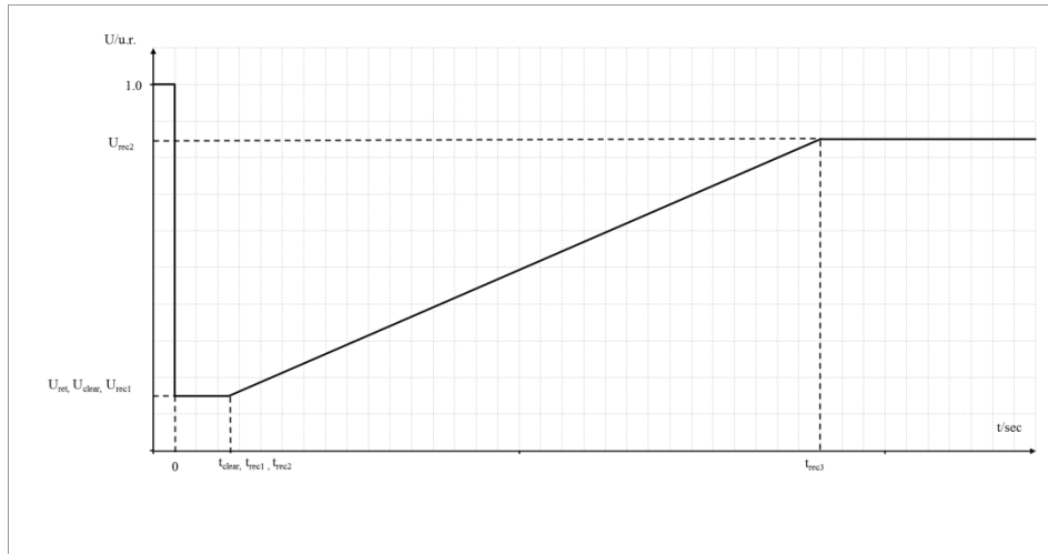
Fig. 3. Diagrama de capabilitate privind trecerea peste defect a IS de categorie B și/sau C
