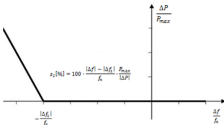
Fig. 5. Capabilitatea de răspuns în putere activă la abaterile de frecvență în modul RFA-SC pentru IS funcționând în regim de producere de energie electrică, unde: P_{max} este referința de putere activă față de care se stabilește \Delta P - și anume puterea maximă a IS; \Delta P este variația puterii active produsă de IS; f_n este frecvența nominală (50 Hz) în rețea și \Delta f este abaterea frecvenței în rețea. În cazul scăderilor de frecvență sub 49,8 Hz, unde \Delta f este mai mic ca -200 mHz, IS funcționând în regim de producere de energie electrică trebuie să crească puterea activă în conformitate cu statismul s_2 .
