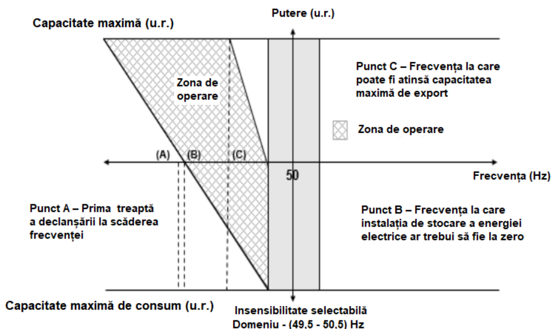
Figura 10 Capabilitatea IS de a trece automat din modul de absorbție de energie din sistem în modul de generare (injecție de putere activă în rețeaua electrică)
