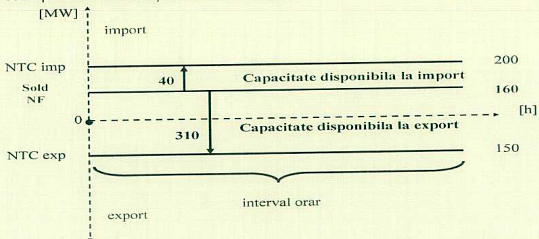
Fig. 2 ATC corespunzătoare direcțiilor de import/export
