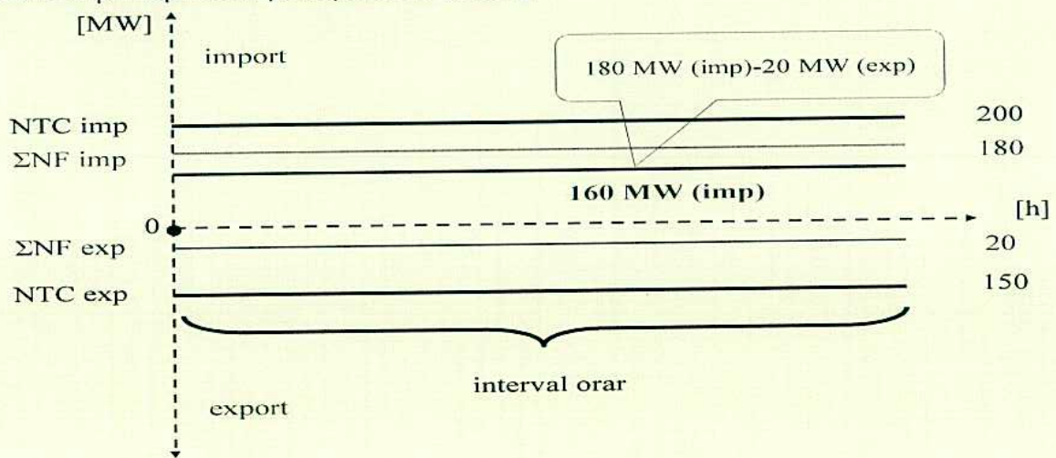
Fig. 1 Soldarea notificărilor (NF) aferente capacităților licitațiilor anterioare celei pentru care se determina ATC prin aplicarea principiului de „netting”
