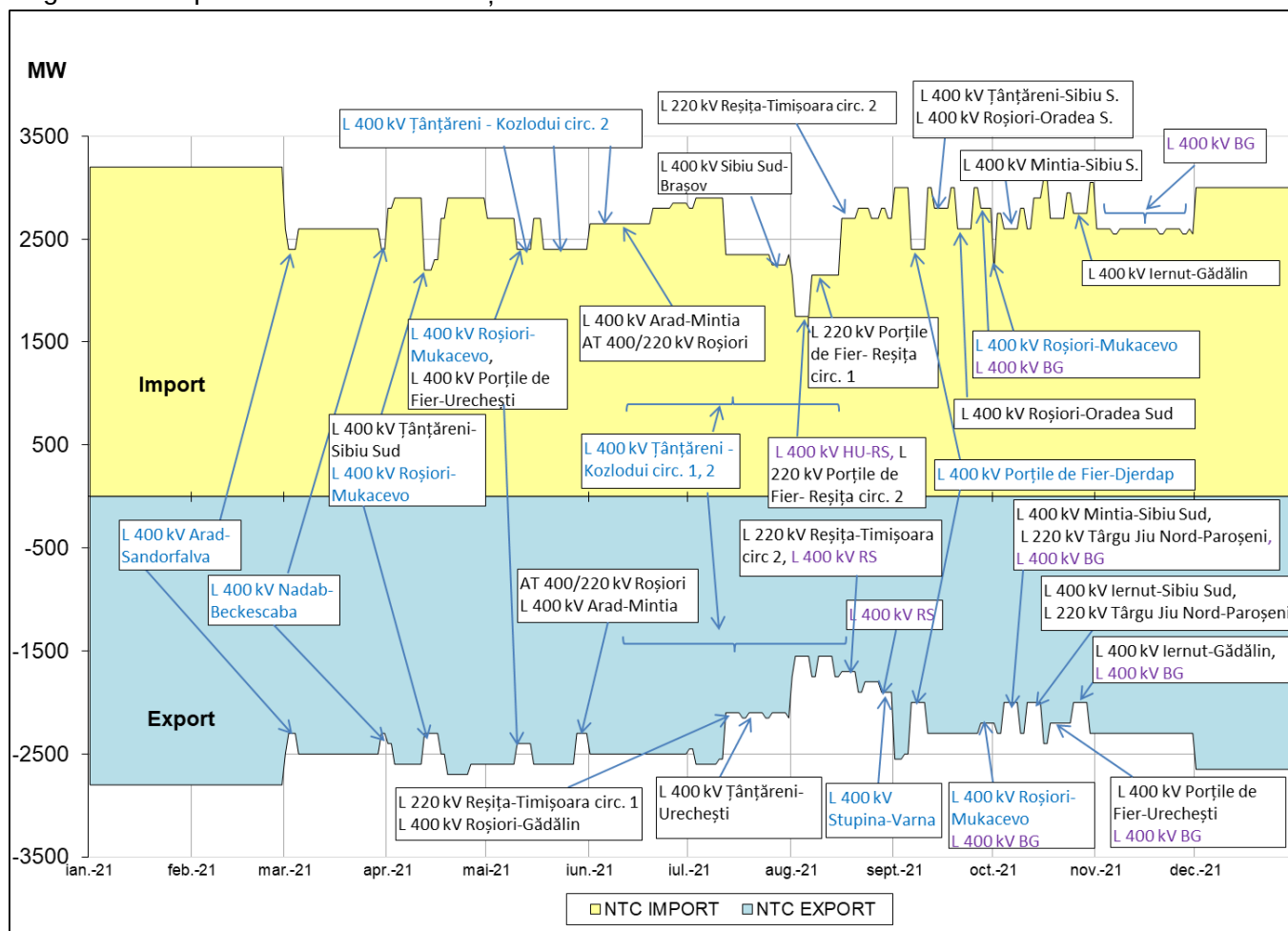
Fig. 4. Retragerile din exploatare care au influențat valorile NTC în anul 2021
