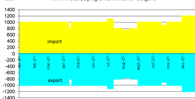
Fig. 2. Profilurile valorilor NTC pe granițe în anul 2021
