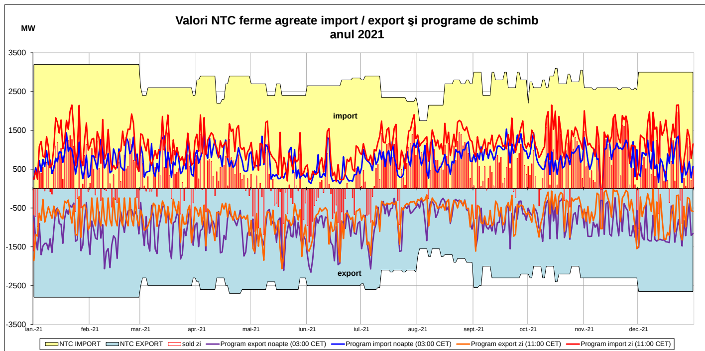
Fig. 3. Valori NTC ferme agreate și programe de schimb pentru anul 2021
