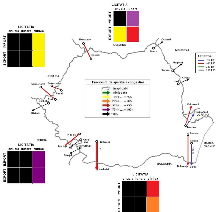
Fig. 1. Frecvența de apariție a congestiei în anul 2021
