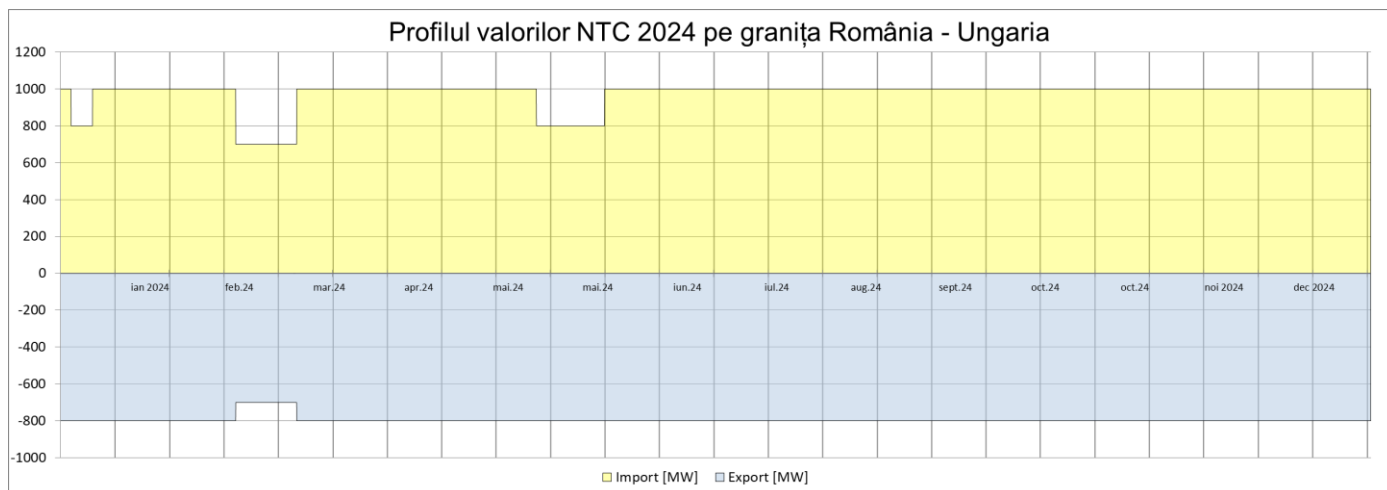
Fig. 3c. Profilul valorilor NTC pe granița România – Ungaria în anul 2024
