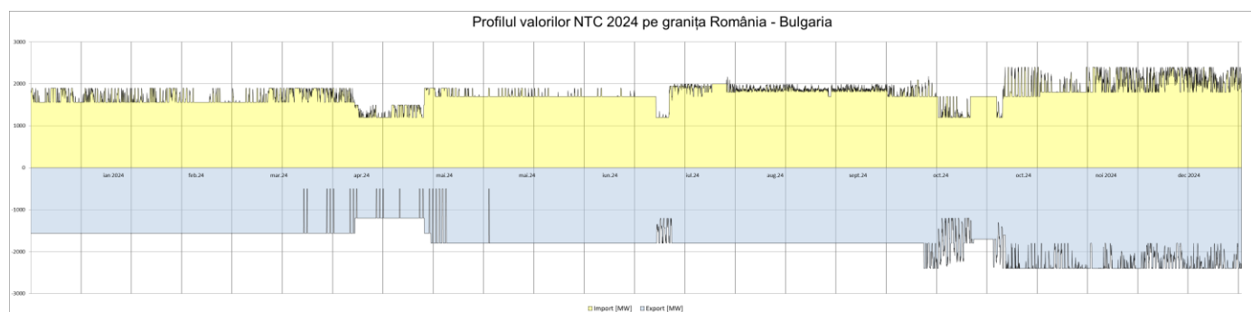
Fig. 3a. Profilul valorilor NTC pe granița România – Bulgaria în anul 2024
