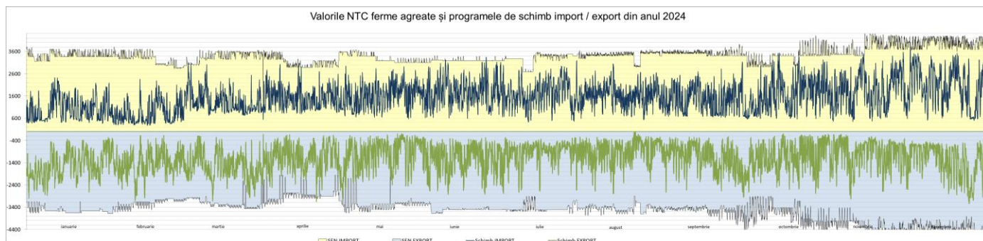
Fig. 4. Valori NTC ferme agreate și programe de schimb pentru anul 2024
