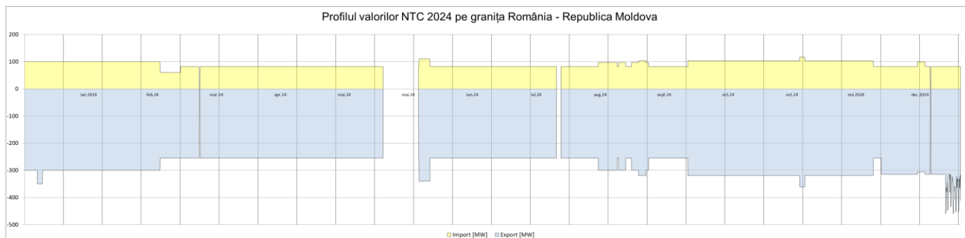
Fig. 3e. Profilul valorilor NTC pe granița România – Republica Moldova în anul 2024
