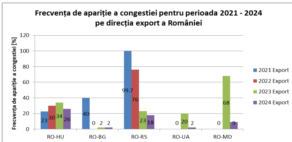
Figura 2a. Frecvența de apariție a congestiei pentru perioada 2021 – 2024, pe granițele SEN unde are loc alocarea de capacitate și pentru direcția export
