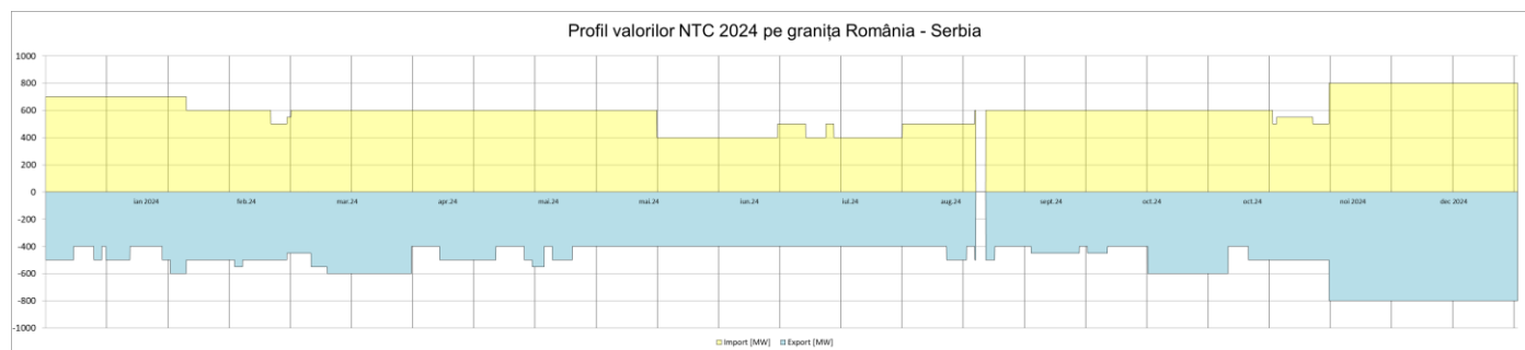
Fig. 3b. Profilul valorilor NTC pe granița România – Serbia în anul 2024
