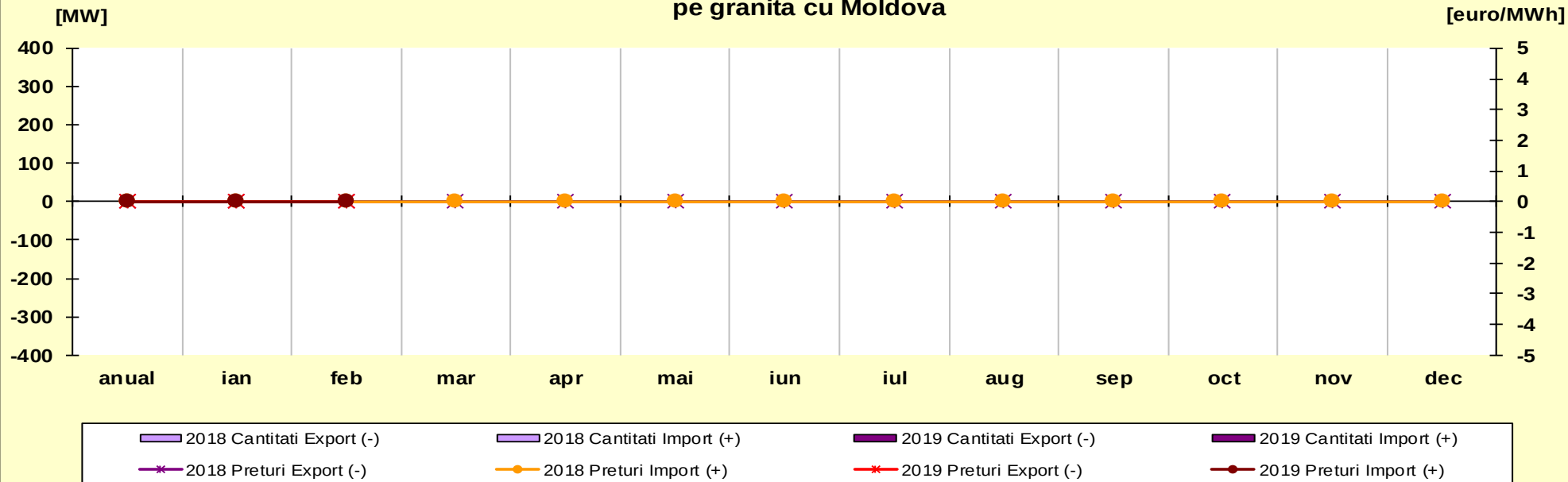
Media Ponderată a Capacitatilor Solicitate corelata cu Pretul de inchidere al Licitatiei, ponderat cu Capacitatea Alocata, pe granita cu Moldova
