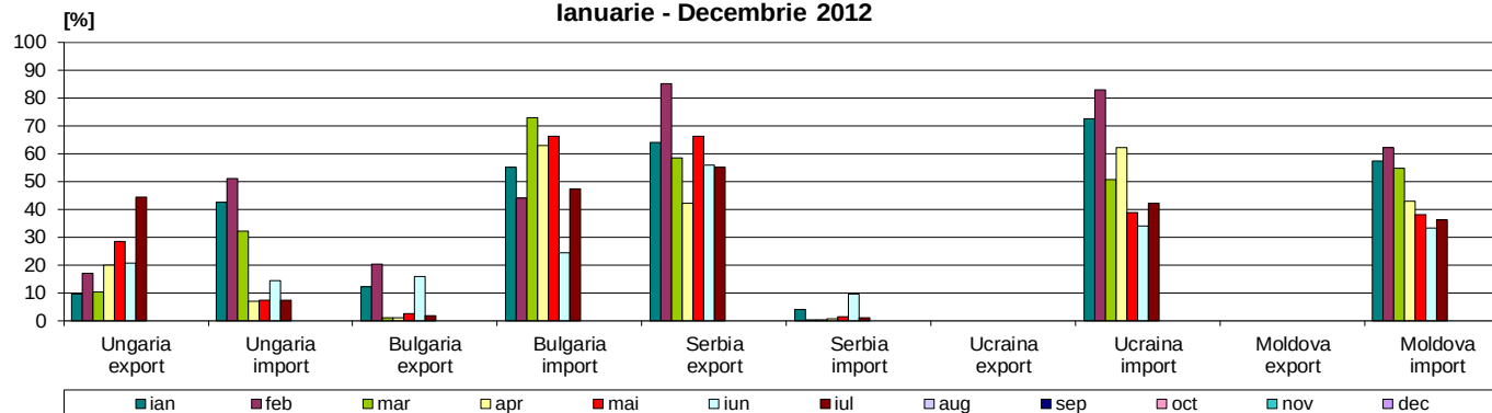
Utilizarea Capacitatii Totale Alocate Ianuarie - Decembrie 2012
